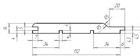
art.010 /Cladding (profile Softline)/Евро (обшивка стеновая) 14x112
