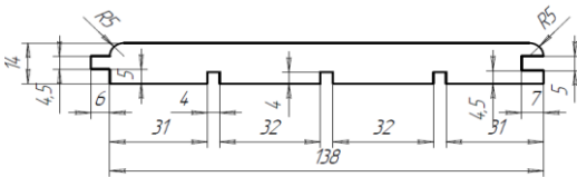
art.017 Cladding (profile Chamfer)/Обшивка стеновая "шпиль" 14x138
