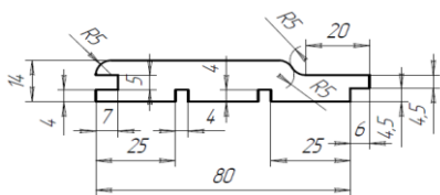
art.009 /Cladding (profile Softline)/Евро (обшивка стеновая) 14x80
