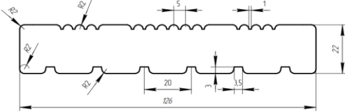
art.021 /Decking (oak)/Террасная доска 22x126
