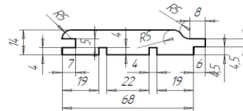
art.008 /Cladding (profile Softline)/Евро (обшивка стеновая) 14x68
