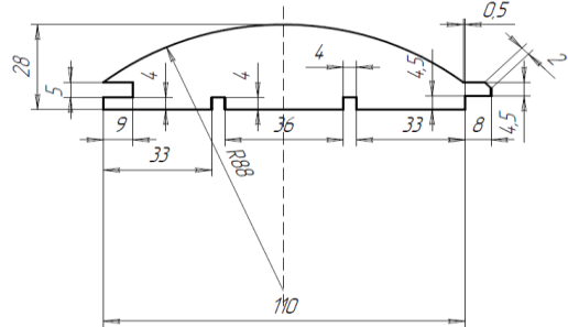
art.002 /Block house/Блок-хаус 28x110
