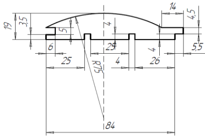
art.001 /Block house/Блок-хаус 19x84
