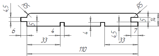
art.018 Handrail/Поручень 60x70
