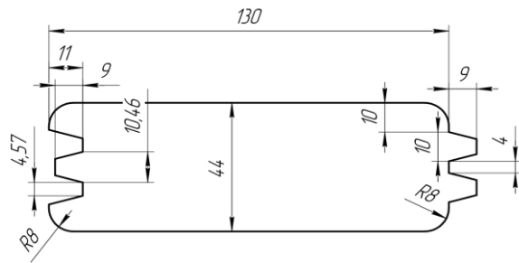
art.004 /Panel/Панель 44x130
