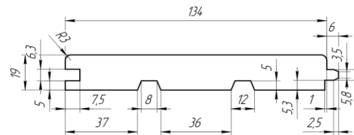
art.020 /Solid wood Flooring (T&G all round)/Массивная паркетная доска (шип-паз с 4-х сторон) 19x134
