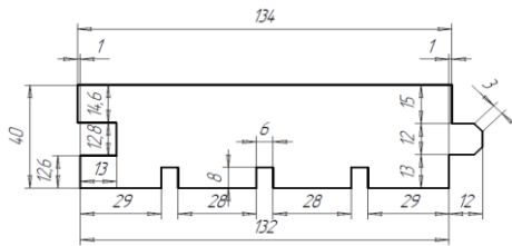
art.007 /Flooring/Доска пола 27/40x134
