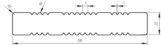
art.022 /Decking (oak)/Террасная доска 22x126
