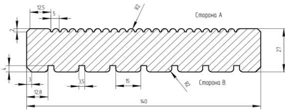
art.003 /Decking (profile Antislip)/Террасная доска "вельвет" 20/27/45x140/145
