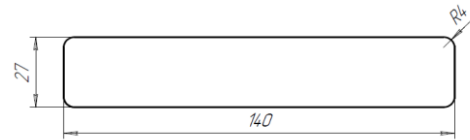
art.014 Decking (profile Smooth)/Террасная доска "гладкая" 20/27/28x120/140
