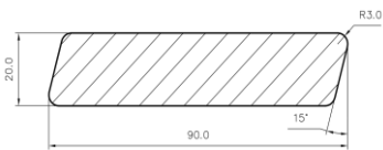
art.005 /Rhombus/Панель 20x68/90
