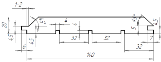
art.011 /Bar imitation/Имитация бруса 20x140
